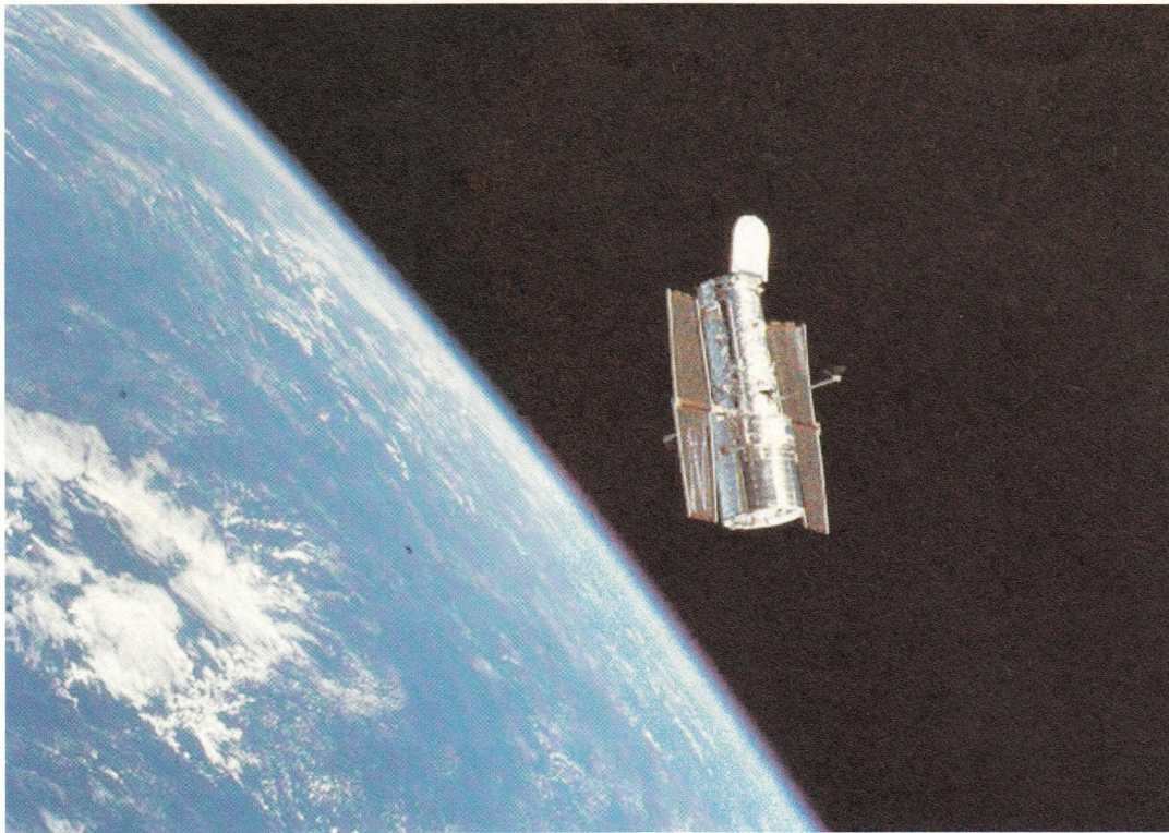
Космический телескоп имени Э. Хаббла, с помощью которого уже открыты планеты других звёзд
